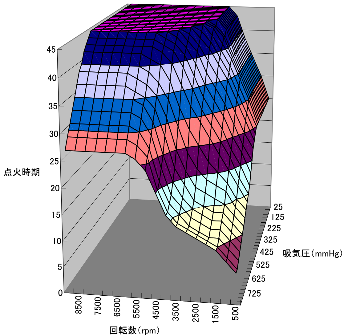
点火マップ
